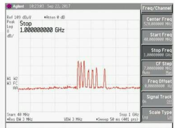
รูปสัญญาณออก
